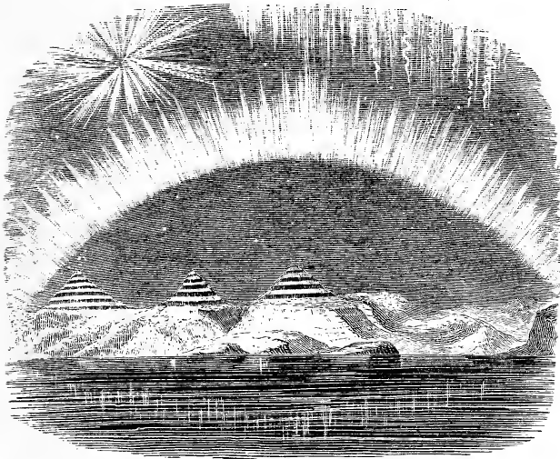
AURORA BOREALIS.
